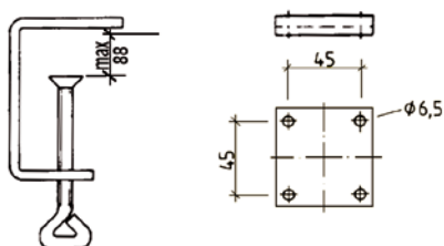
Tischklemme (TK)/Table clamp (TK) Pince de fixation (TK)/Pinza de fijación (TK)
