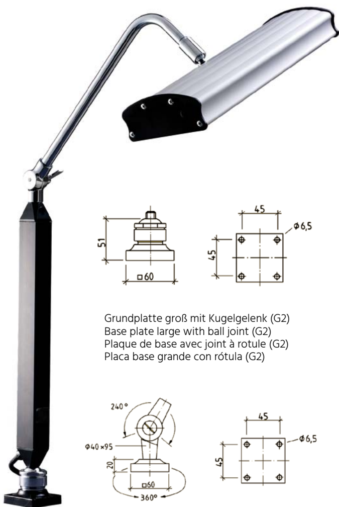
Grunddrehplatte mit Kippgelenk (GD) Rotary base plate with tilting joint (GD) Plaque giratoire avec joint basculant (GD) Placa base con rótula con dispositivo basculante (GD)
