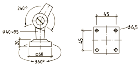
Grunddrehplatte mit Kippgelenk (GD) Rotary base plate with tilting joint (GD) Plaque giratoire avec joint basculant (GD) Placa base con rótula con dispositivo basculante (GD)
